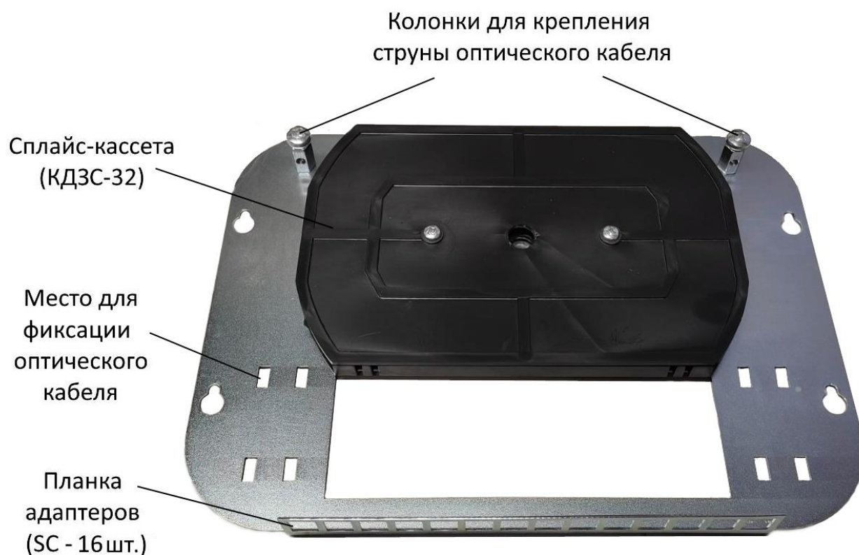
Рисунок 3.3 - Оптический кросс.
