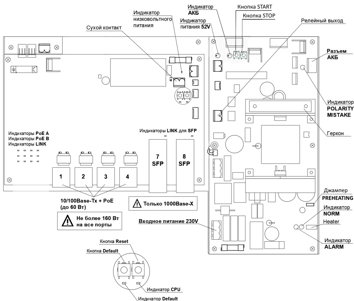
Рисунок 3.4.2 – Расположение элементов PSW-2G+UPS-Box
