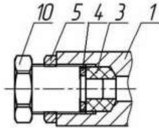
ЗГ, заглушка для отверстия под кабельный ввод
