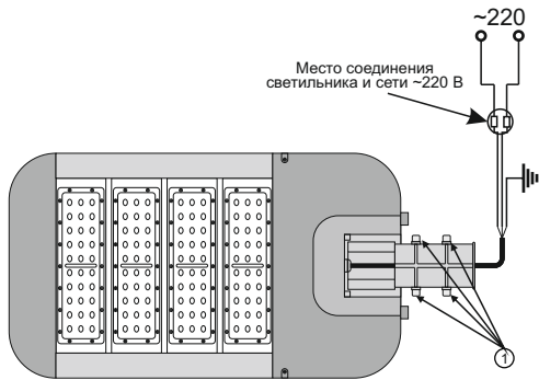
Рисунок 2 — Схема подключения изделия
