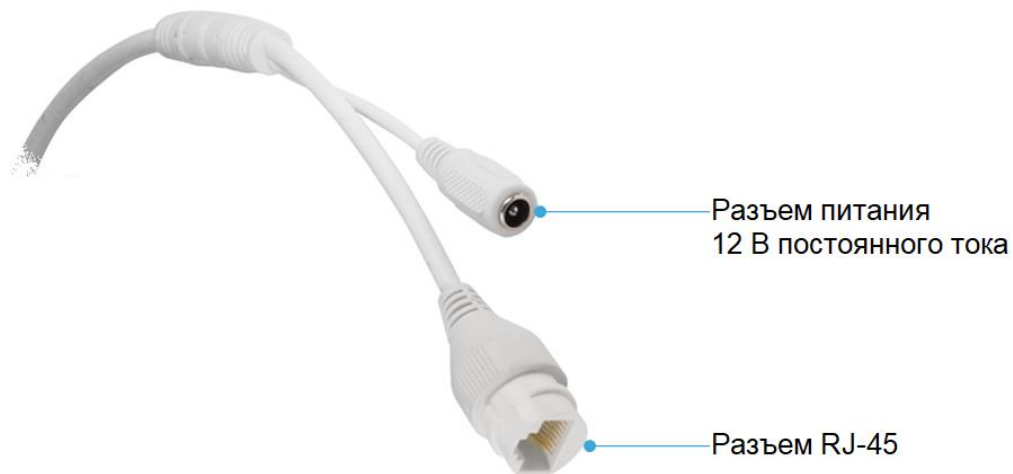
Рисунок 6.1 – Кабель видеокамеры
