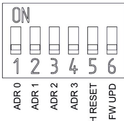
Рисунок 4. 6 Назначение DIP-переключателей
