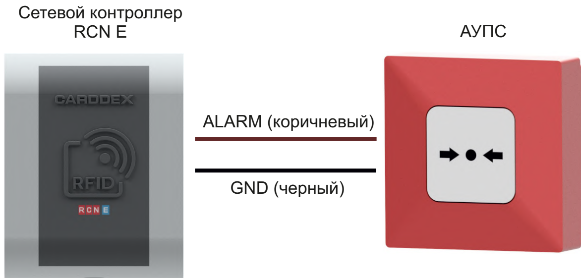
Рисунок 4.2 Подключение к «RCN E» АУПС
