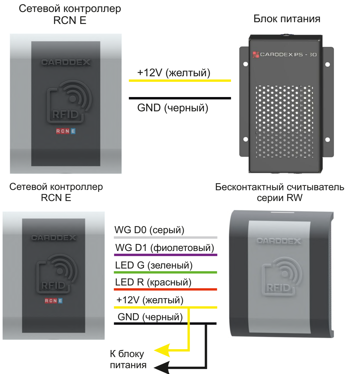
Рисунок 4.1 Подключение контроллера и считывателя к питанию
