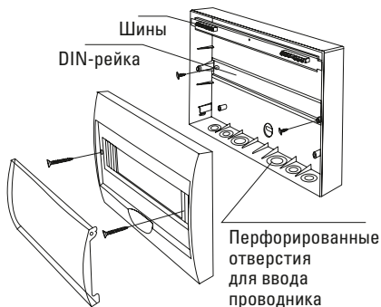
Рис. 1 - Схема монтажа ЩРН-П
