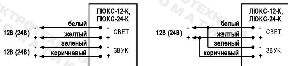
Рис.1. Схема подключения.
