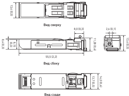
Рис. 1 — Габаритные размеры TSX-SFP-HS1D-15-20
