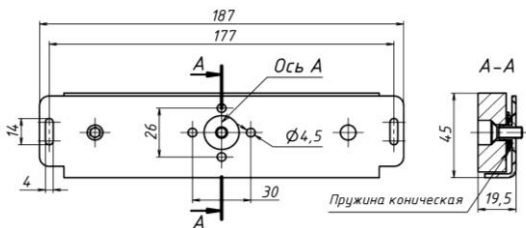
Рисунок 3 - Якорная часть
