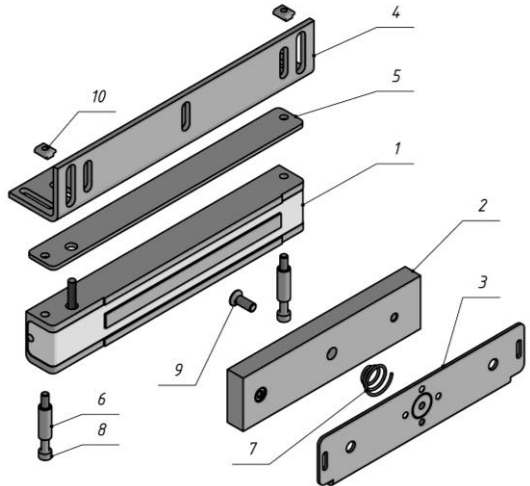
Рисунок 1 – Комплект поставки замка ALM-300FP
