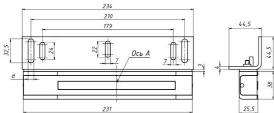
Рисунок 2 - Корпусная часть
