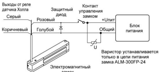
Рисунок 4 - Схема подключения замка ALM-300FP
