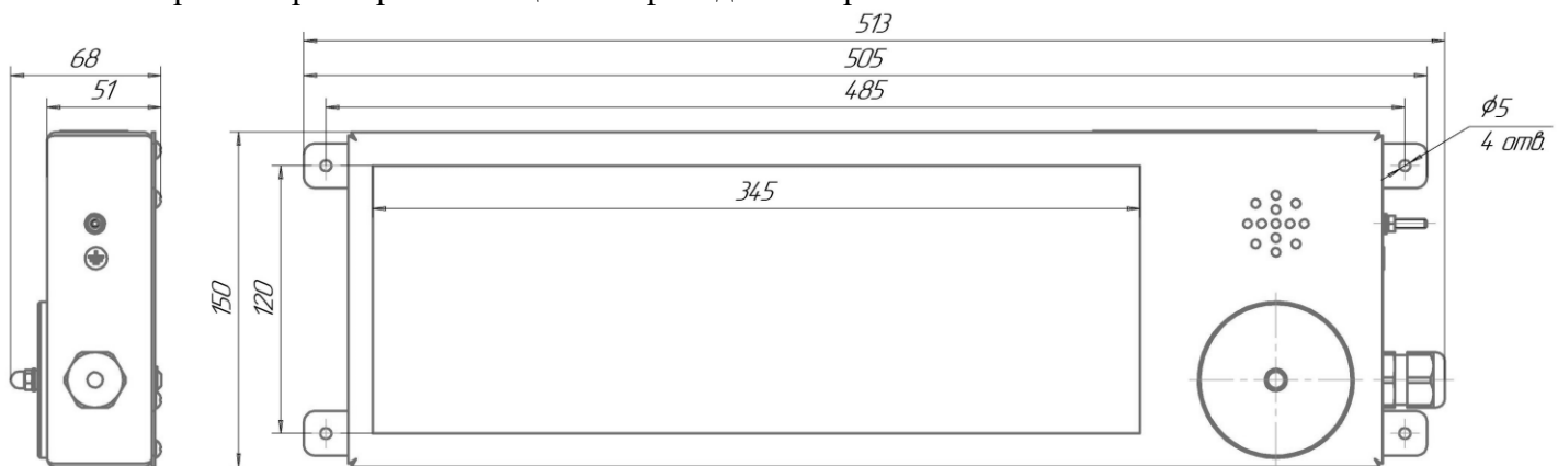
Рис. 1 – Оповещатель пожарный взрывозащищенный комбинированный
