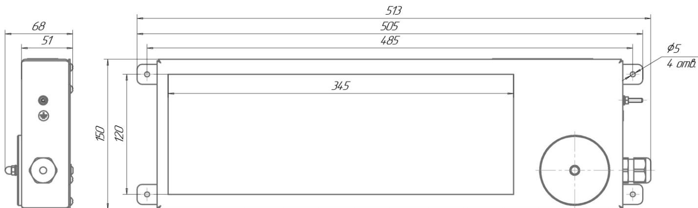
Рис. 2 – Оповещатель пожарный взрывозащищенный световой
