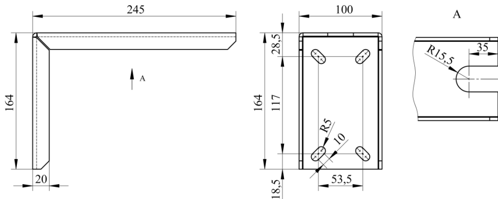
Рисунок 4.14- Кронштейн крепления настенный вертикальный типа КРНВ.І - 20
