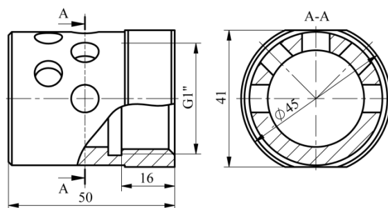
Рисунок 4.6 - Насадок настенного типа с распылом ГОТВ на 180° для модуля типа «Импульс-20-Т»
