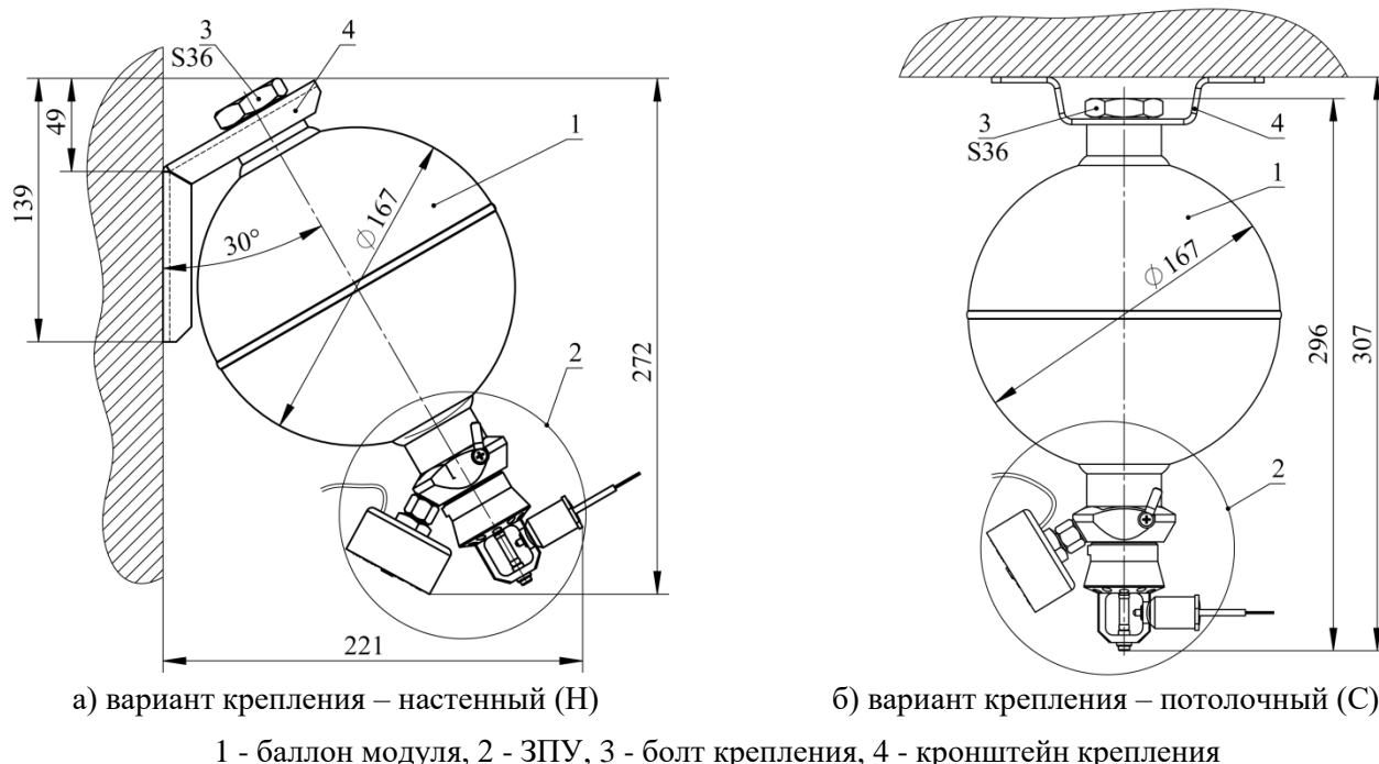
Рисунок 4.1 - Общий вид модуля типа «Импульс-2»
