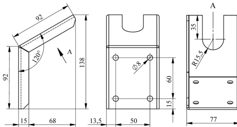
Рисунок 4.11- Кронштейн крепления настенный типа КРН.І - 2
