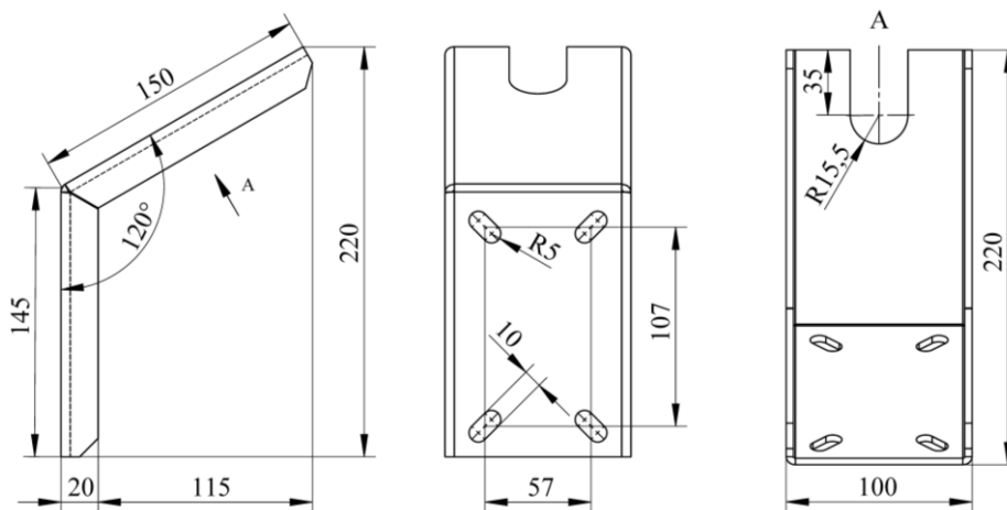
Рисунок 4.12- Кронштейн крепления настенный типа КРН.І - 20
