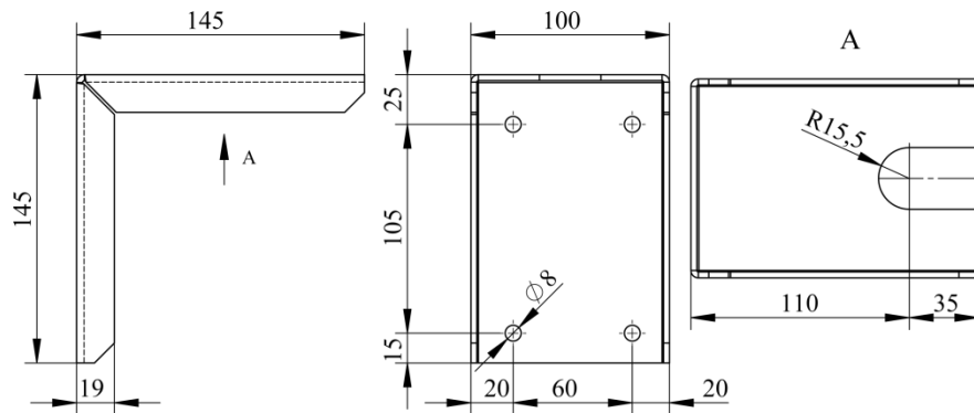
Рисунок 4.13- Кронштейн крепления настенный вертикальный типа КРНВ.І - 2
