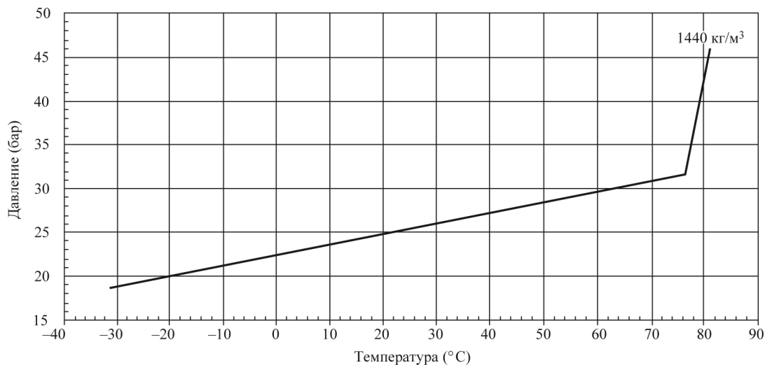
Рисунок А.3 - График зависимости давления в баллоне модуля от температуры для огнетушащего состава FK-5-1-12 при различных коэффициентах заполнения
