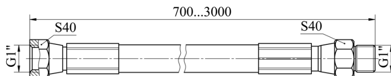
Рисунок 4.8- Рукав высокого давления типа PVT – 25
