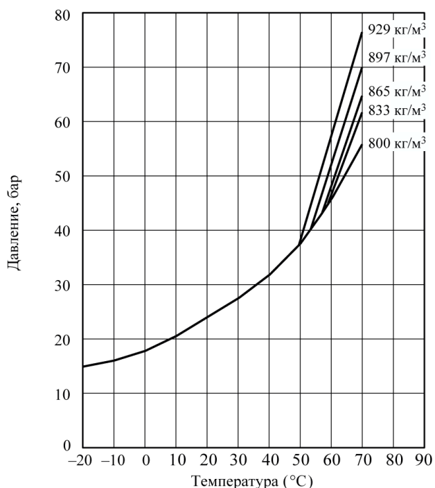
Рисунок А.1 – График зависимости давления в баллоне модуля от температуры для огнетушащего состава НС 125 при различных коэффициентах заполнения
