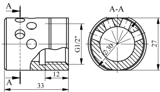
Рисунок 4.4 – Насадок настенного типа с распылом ГОТВ на 180° для модуля типа «Импульс-2-Т»
