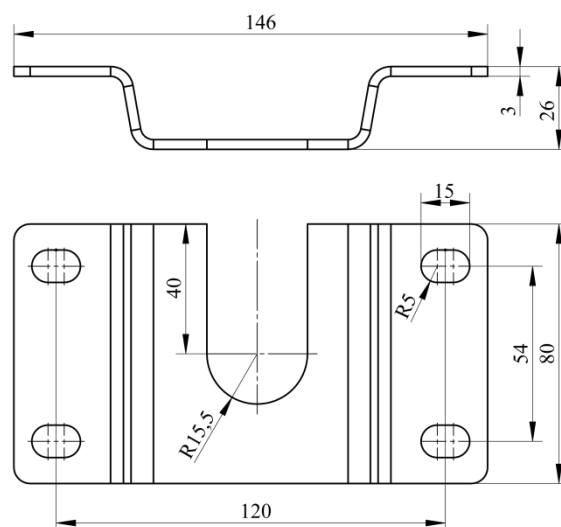
Рисунок 4.9– Кронштейн крепления потолочный типа КРС.І – 2
