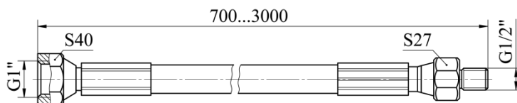
Рисунок 4.15– Рукав высокого давления типа РВД – 16
