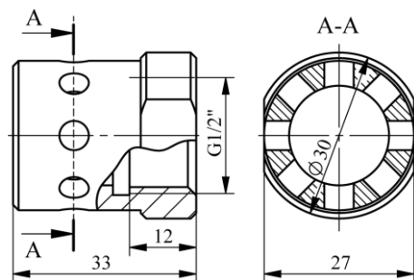
Рисунок 4.5 – Насадок потолочного типа с распылом ГОТВ на 360° для модуля типа «Импульс-2-Т»
