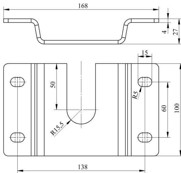
Рисунок 4.10- Кронштейн крепления потолочный типа КРС.І - 20
