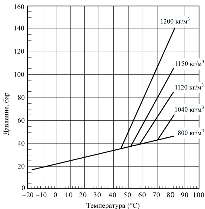
Рисунок А.2 - График зависимости давления в баллоне модуля от температуры для огнетушащего состава НС 227еа при различных коэффициентах заполнения
