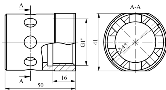
Рисунок 4.7 - Насадок потолочного типа с распылом ГОТВ на 360° для модуля типа «Импульс-20-Т»
