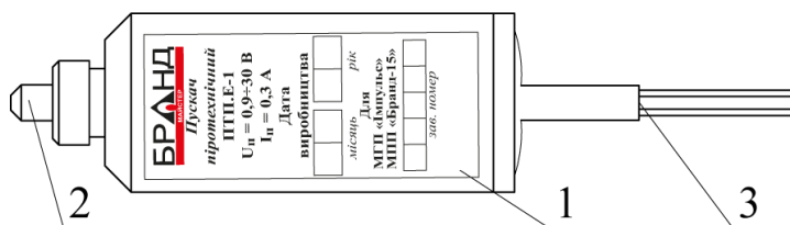
Рисунок 4.3– Пиротехнический пускатель
