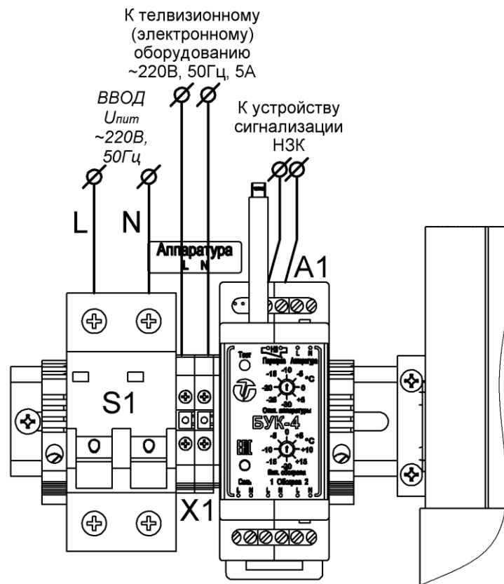
Рис. 2. Подключение термошкафа
