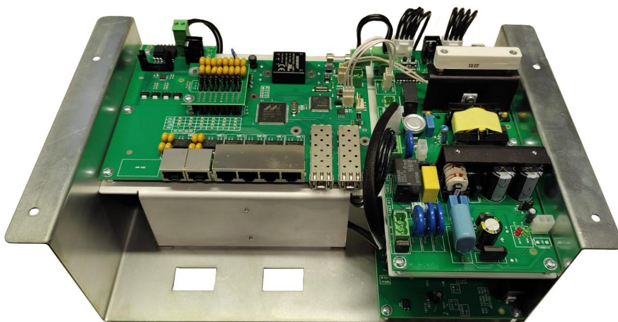
Рисунок 3.4.1 - Платы коммутатора и блоков питания
