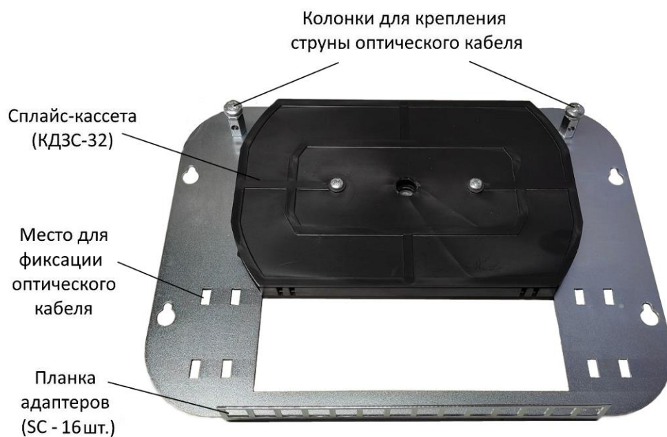
Рисунок 3.3 - Оптический кросс.
