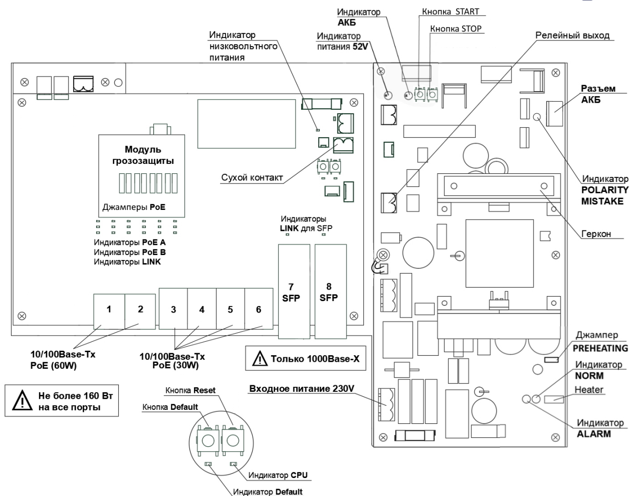
Рисунок 3.4.2 – Расположение элементов PSW-2G6F+UPS-Box
