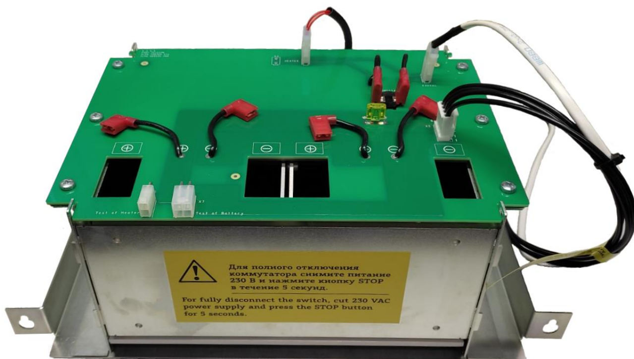
Рисунок 3.6 – отсек АКБ.
