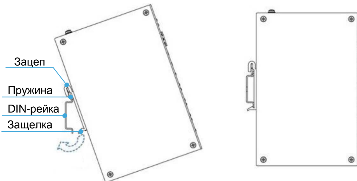
Рисунок 5.3 – Инсталляция
