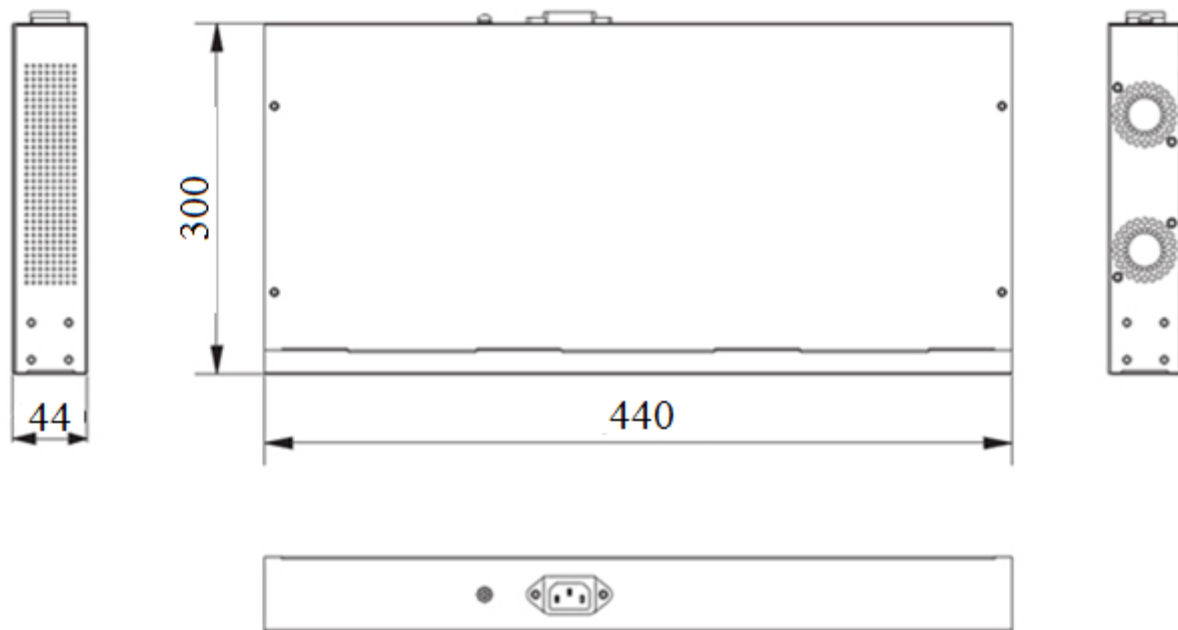
Рисунок 2 – Габаритные размеры
