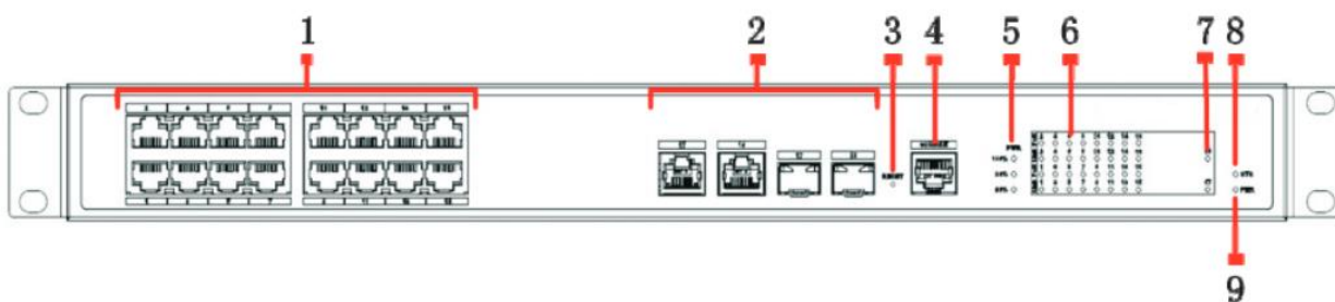
Рисунок 1 – Передняя панель
