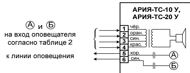
Рис.1. Схема подключения.
