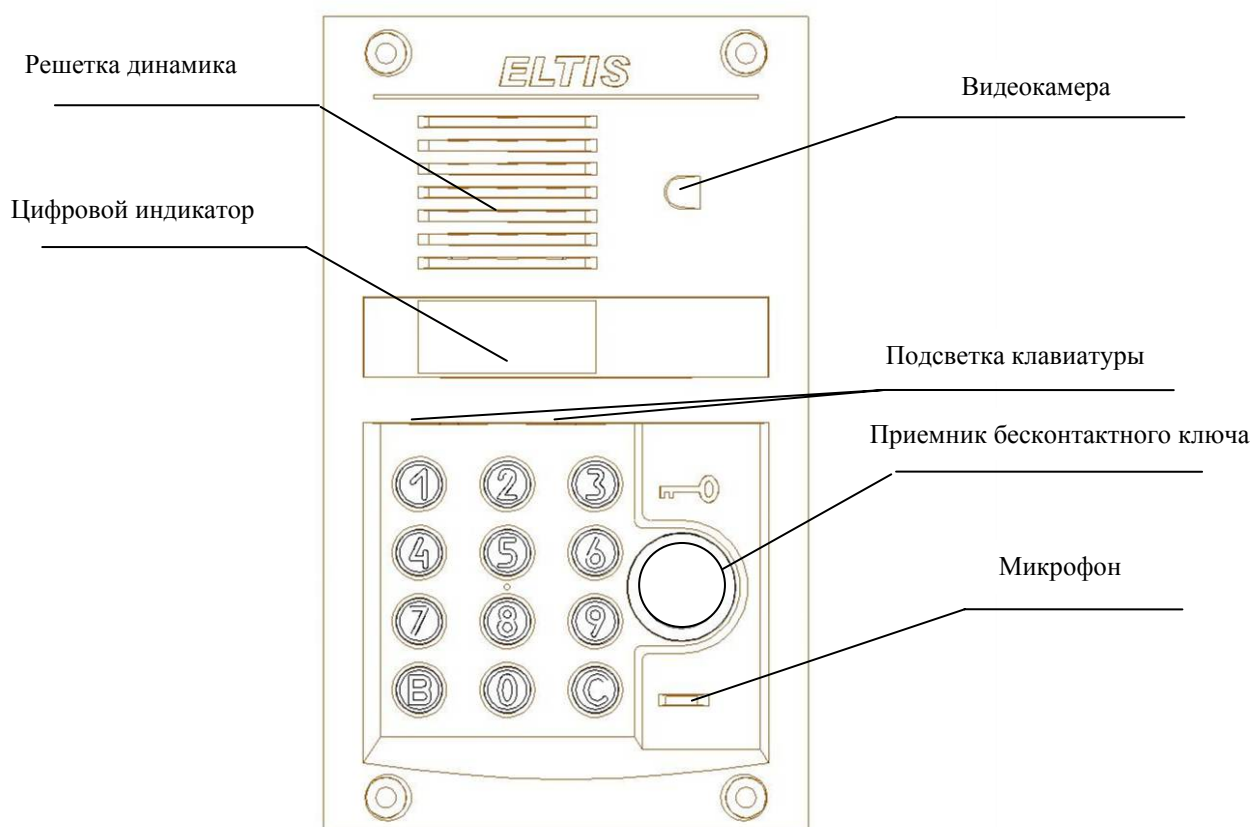
Рис.1 Внешний вид со стороны лицевой панели блока вызова DP300-RDV24.
