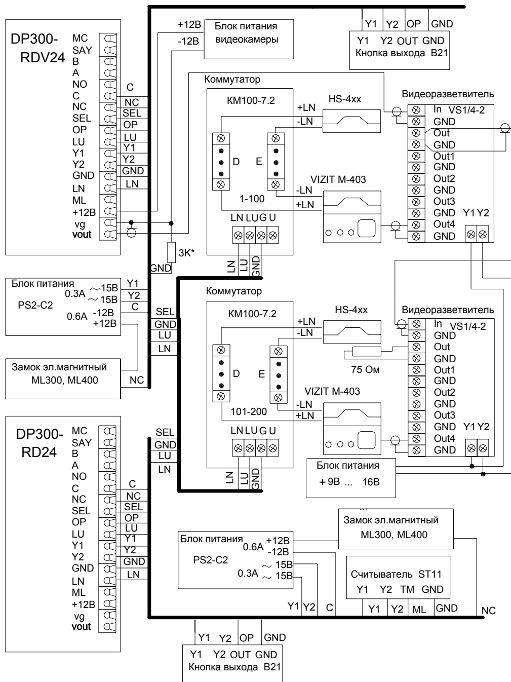
Рис.3 Пример схемы подключения DP300-RDV24 в составе домофонного комплекса.
