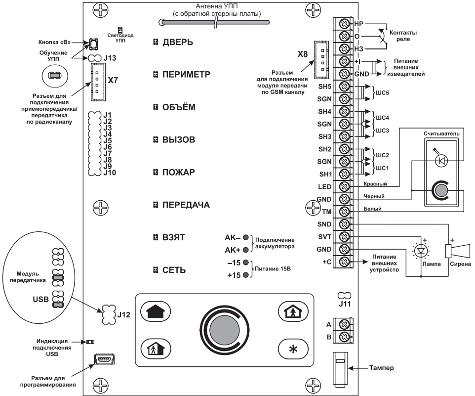
Рисунок 11 – Монтажная схема охранной панели
