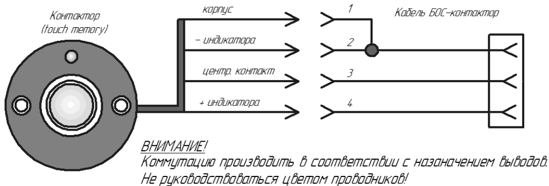
Рисунок 2.4 – Схема подключения контактора
