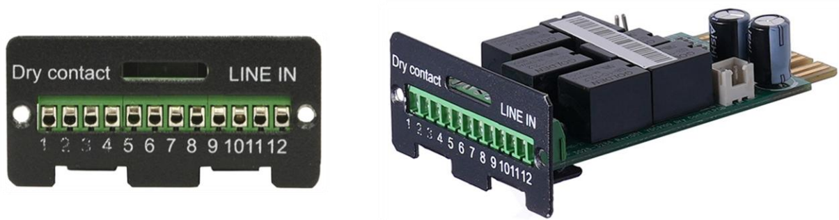
Внешний вид мини карты релейного интерфейса
