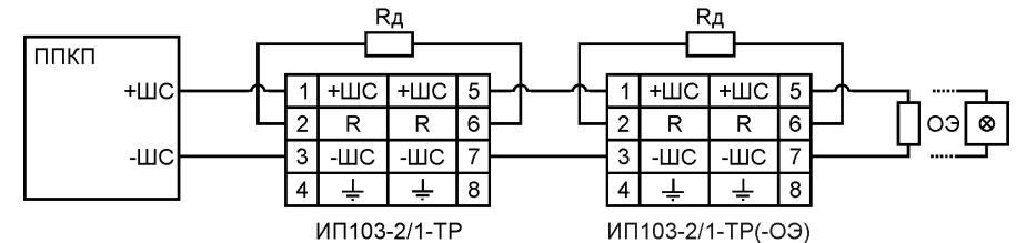
Рисунок 7. Пример схемы подключения извещателей в шлейф сигнализации.
