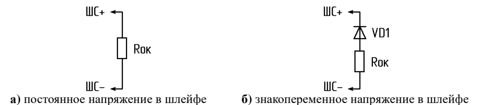
Рисунок 8. Оконечный элемент контроля шлейфа ППКП.
