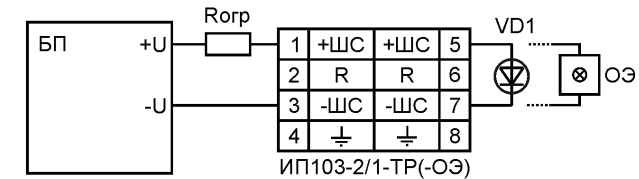
Рисунок 5. Схема электрическая извещателя.
