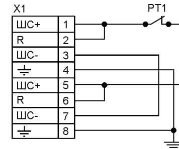
Рисунок 5. Схема электрическая извещателя.
