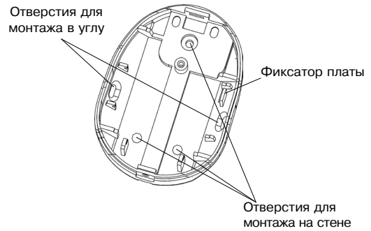
Рисунок 2 – Основание извещателя
