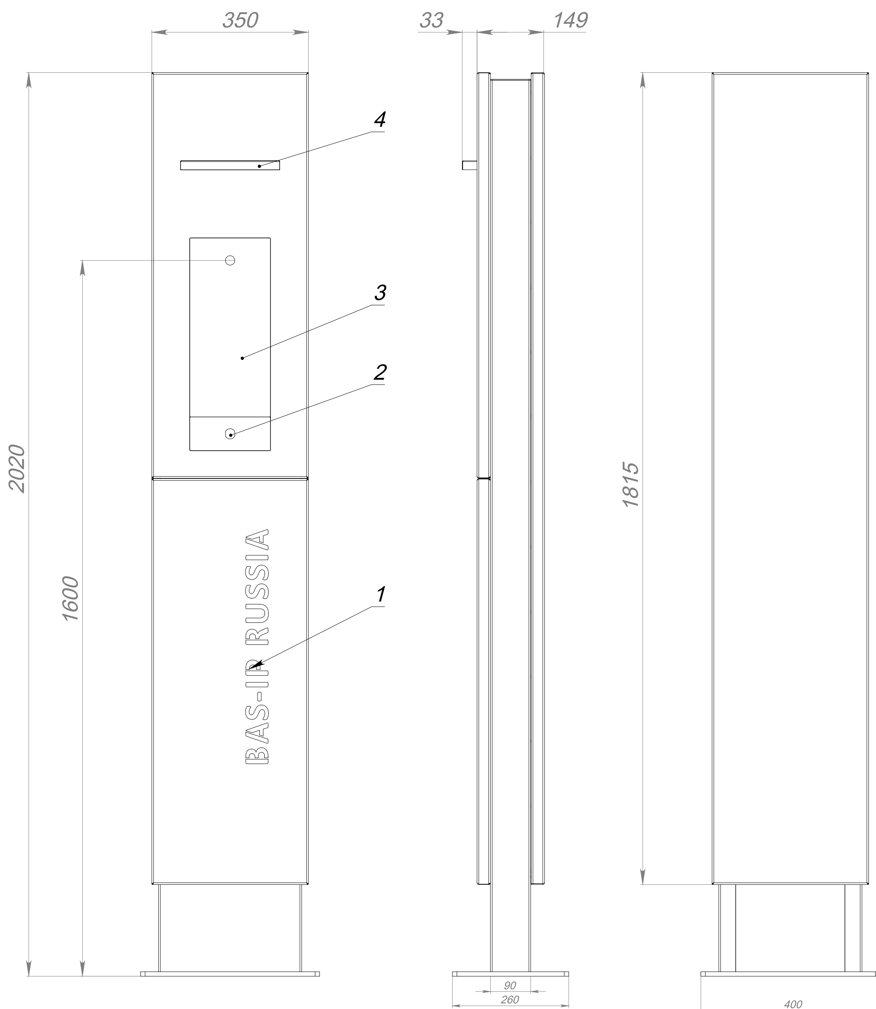
Рис.1 Внешний вид, габаритные размеры
