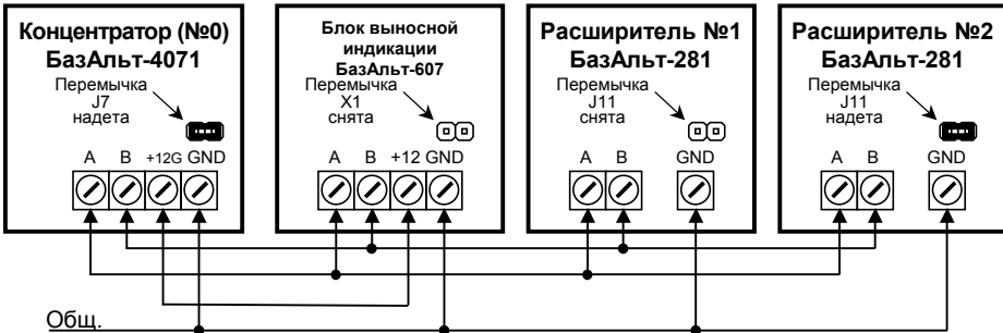
Рисунок 9 – Пример подключения расширителей к концентратору
