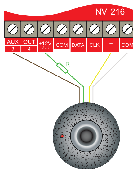
Считыватель СТМ-КТ
