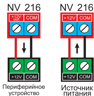
Рисунок 1. Подключение питания
