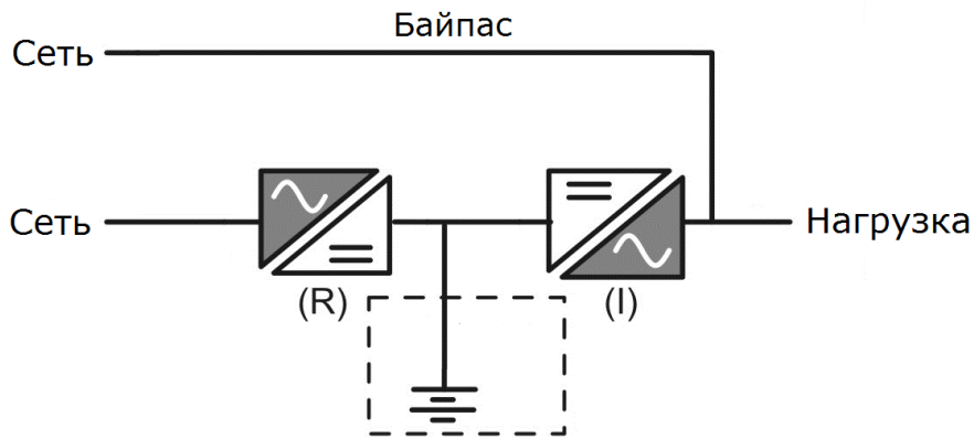
Рисунок 2 - Блок-схема
