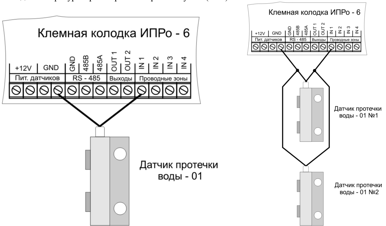
Подключение 1 датчика
