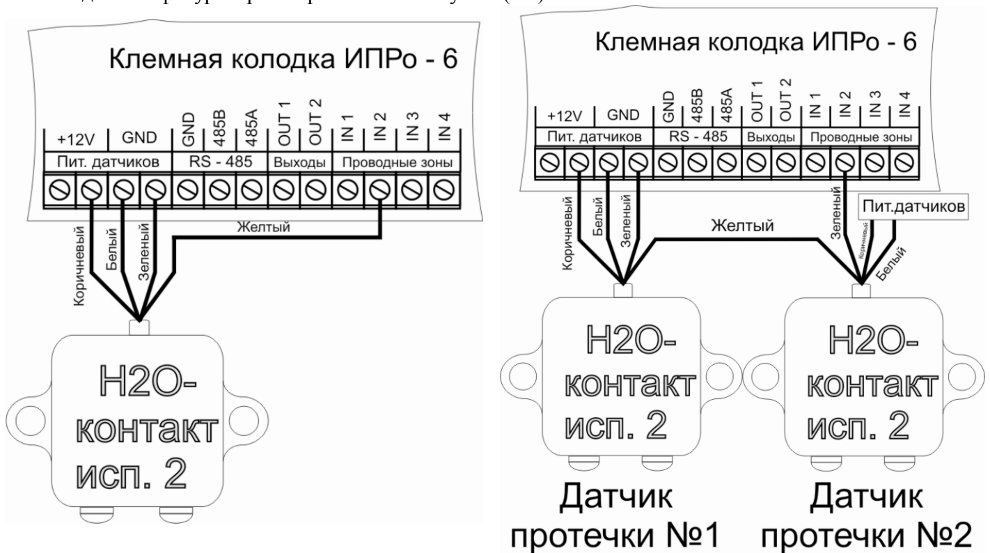
Подключение 1 датчика
