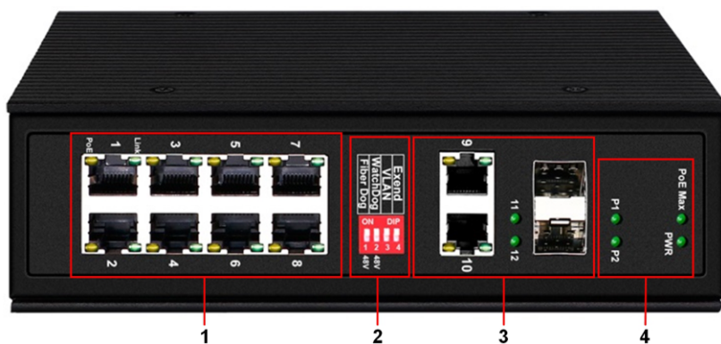
Рис.1 Разъемы и индикаторы на передней панели NS-SW-8G4G-P/I
