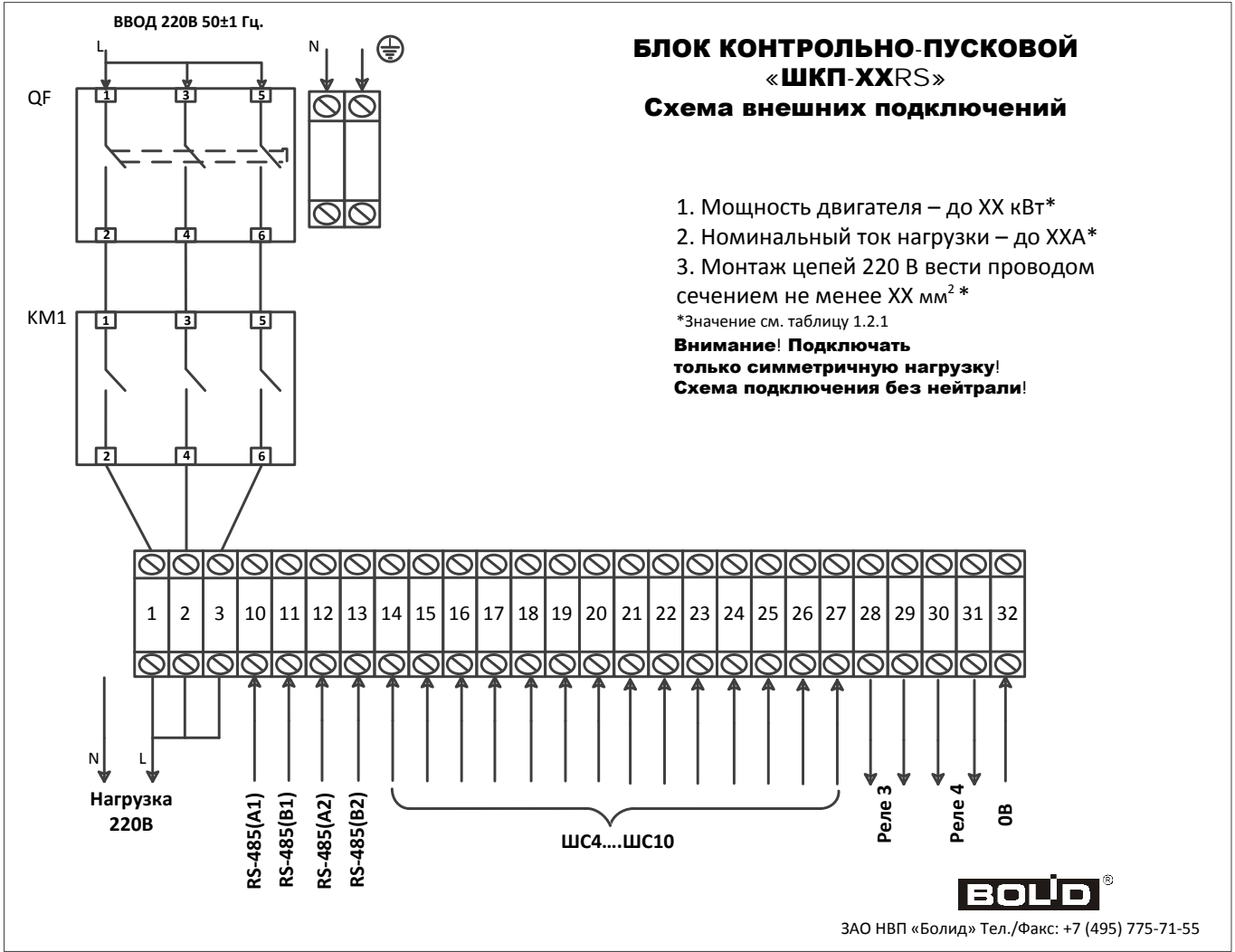
Рисунок 3в. Схема подключения блоков ШКП-4-10-18-30RS при 220В.
