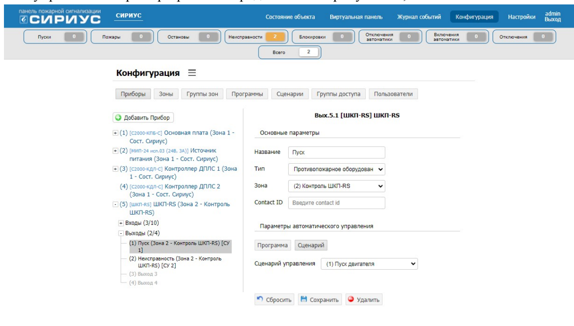
Рисунок 9а. Привязка программ управления к первому выходу блока.
