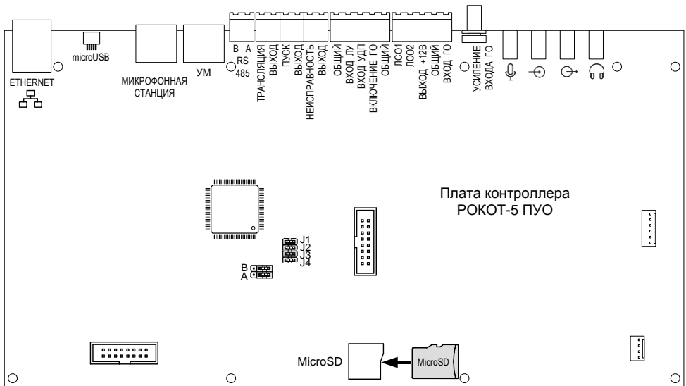
Рис.А7 Внешний вид платы контроллера ПУО (интерфейс RS-485 в данной версии ПУО не используется)
