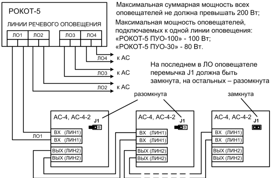
Рис.А3 Схема подключения «АС-4» и «АС-4-2» к линиям оповещения
