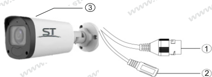
Рис.1 Схема подключения видеокамеры
