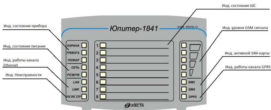
Рисунок 2.4. Панель индикации ППКОП «Юпитер IP/GPRS»
