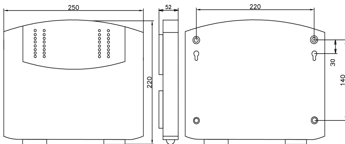
Рисунок 4.1. Габаритные и установочные размеры прибора, пластмассовый корпус
