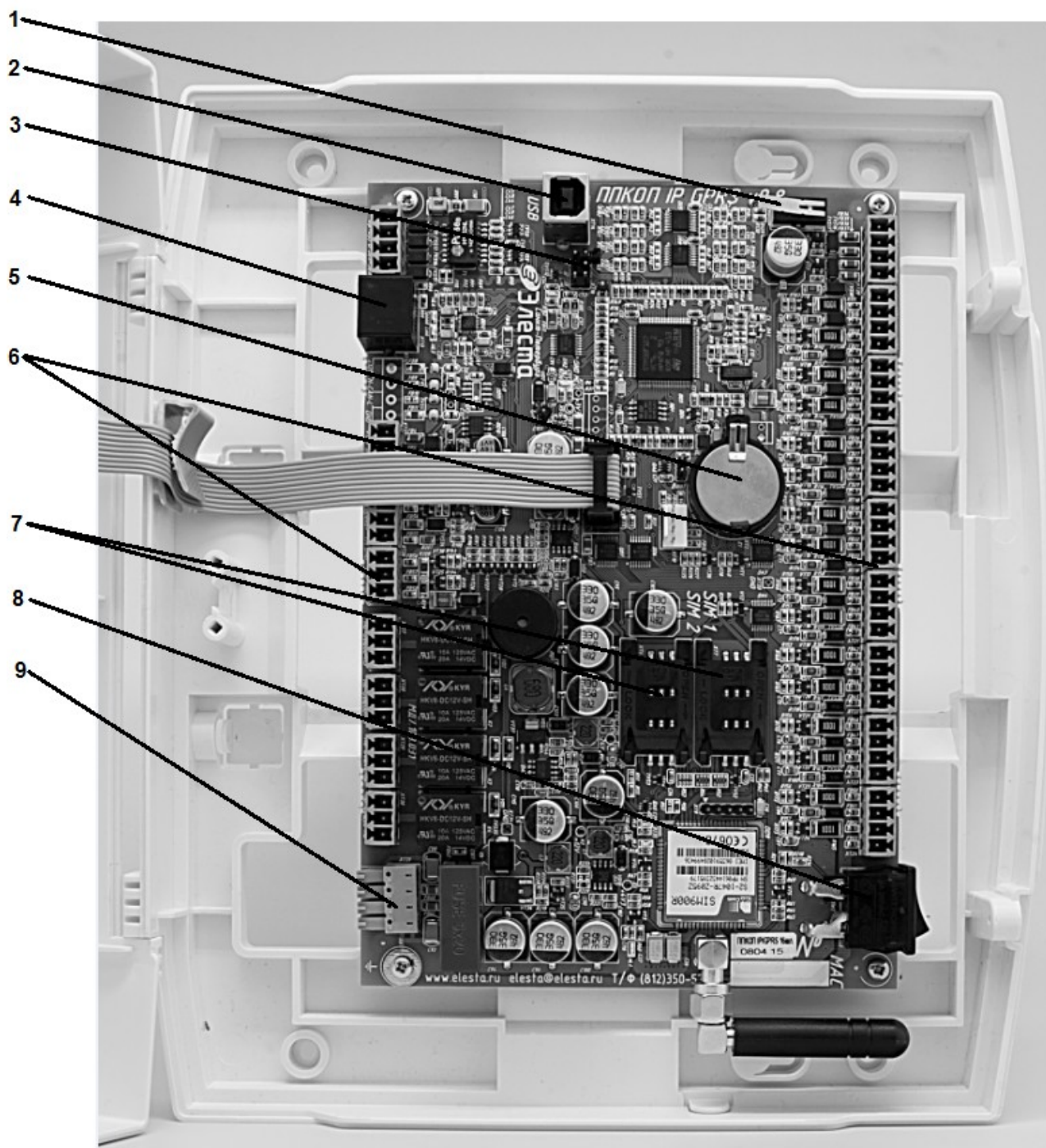
Рисунок 2.3. Вид прибора с открытой крышкой
