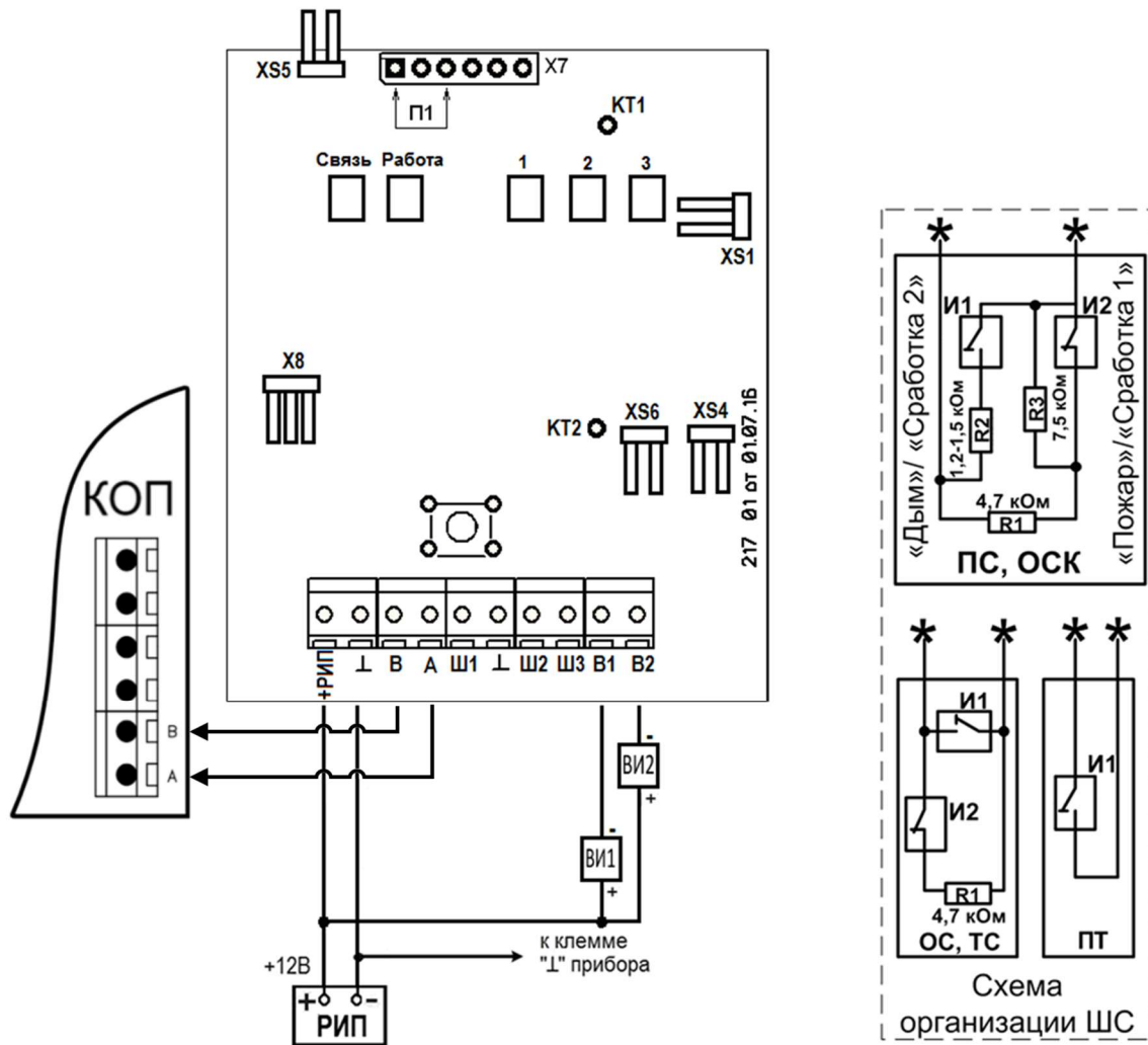
Рисунок 14 – Схема подключения
