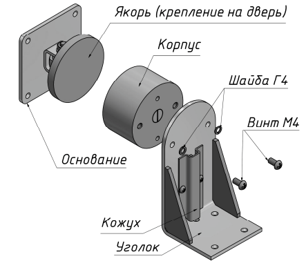
Рисунок 2 – Крепление корпуса замка на L-уголок
