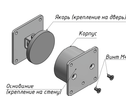
Рисунок 1 – Комплект поставки замка AL-50FC
