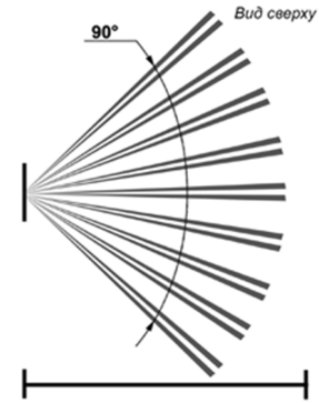
«Фотон-20» (15 м) «Фотон-12» (12 м) «Фотон-12-1» (12 м) «Фотон-12-РК» (12 м)
