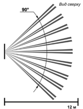
«Фотон-10М» «Пиرون-4» «Фотон-10М-01» «Пиرون-4» исп.1 «Фотон-10МД» «Пиرون-4» исп.2 (18 м) «Орлан» «Пиرون-7»
