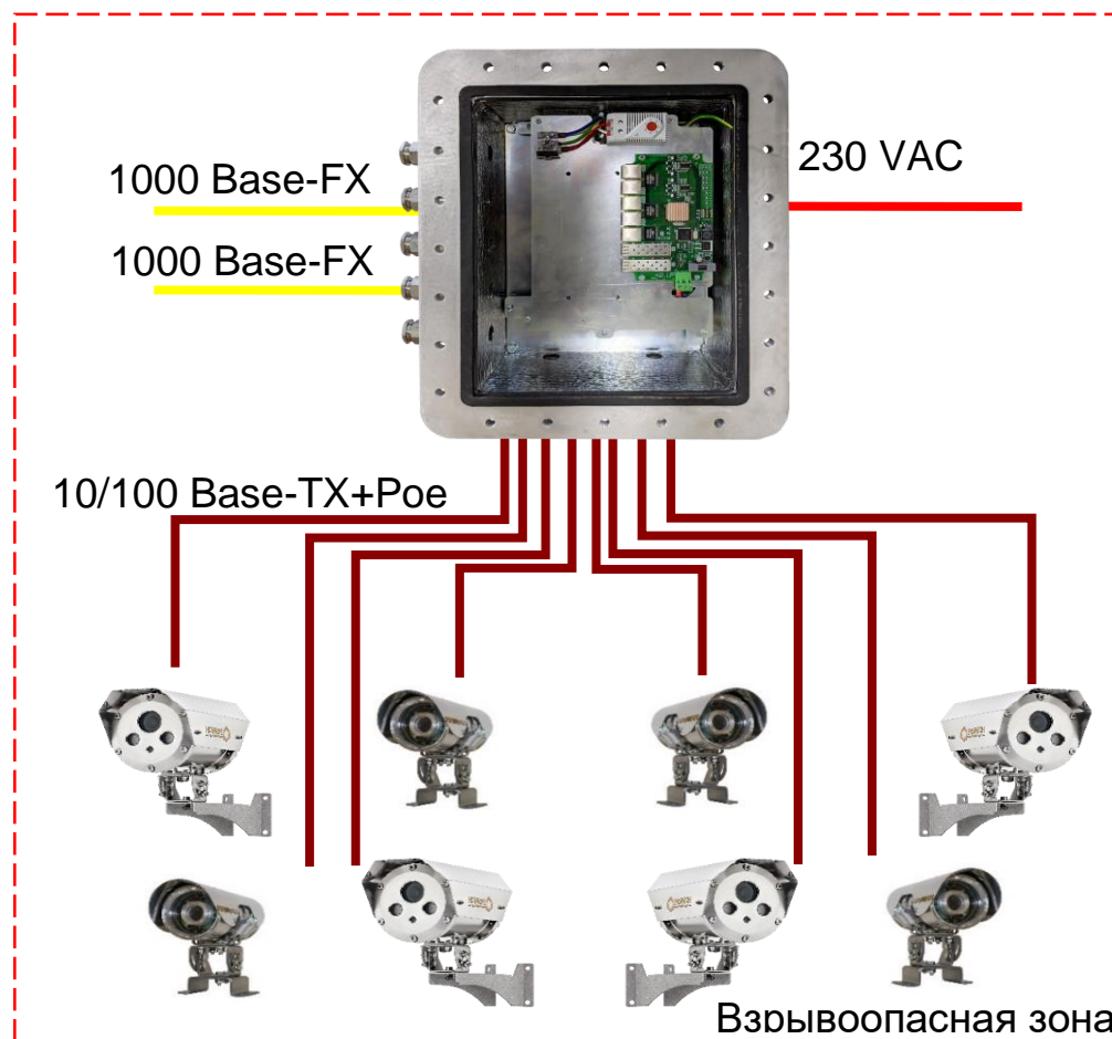
Рисунок 2. Типовая схема подключения коммутатора по двум оптическим кабелям.
