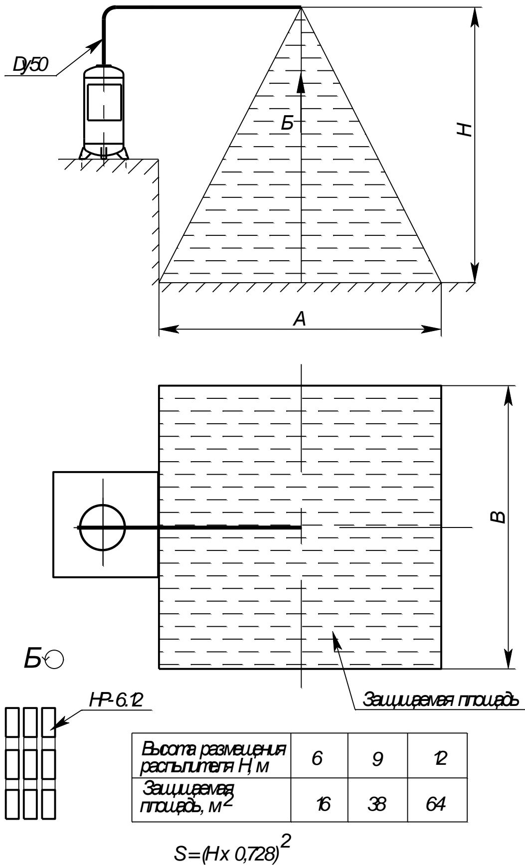
Рис. А9 - Конфигурация защищаемой площади модуля с насадком-распылителем HP-6.12 (варианта размещения 8)
