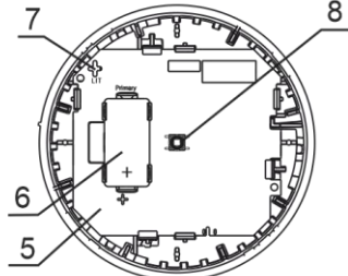
Электронный блок Вид снизу
