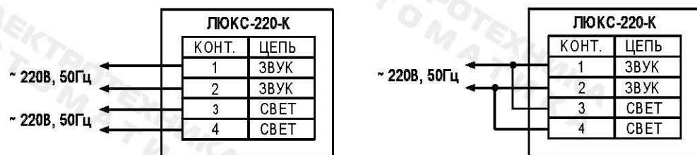
Рис.1. Схемы подключения.
