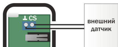
Рисунок 5.5 – Схема подключения внешнего проводного датчика открытия
