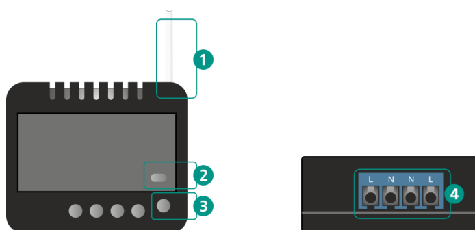
Рисунок 2.14 – Внешний вид реле Livi Relay и Livi Relay 12/24
