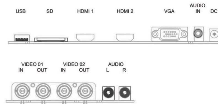
Рис. 1 Схема расположения и назначение разъемов.
