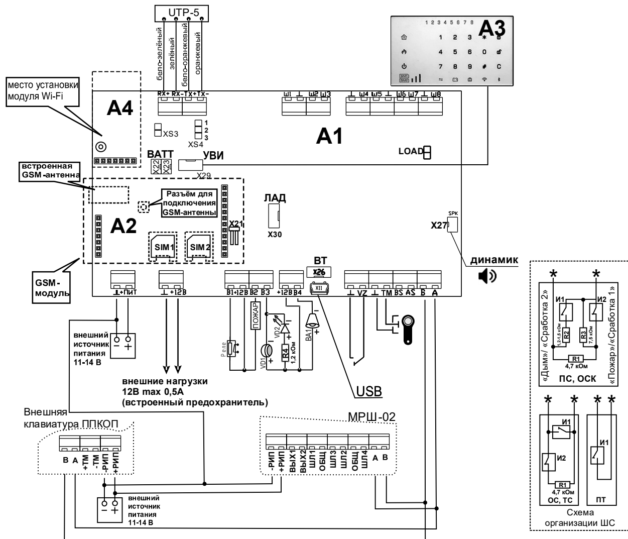
Рисунок 6 – Схема подключения прибора версии Приток-А-КОП-04
