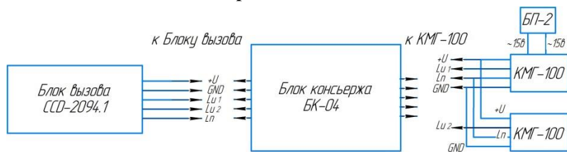
Рис. 1 Структурная схема соединения устройств с БК-04
