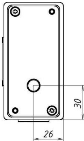
Рисунок 4 – Установочные размеры считывателя ALM-PROX (вариант W)
