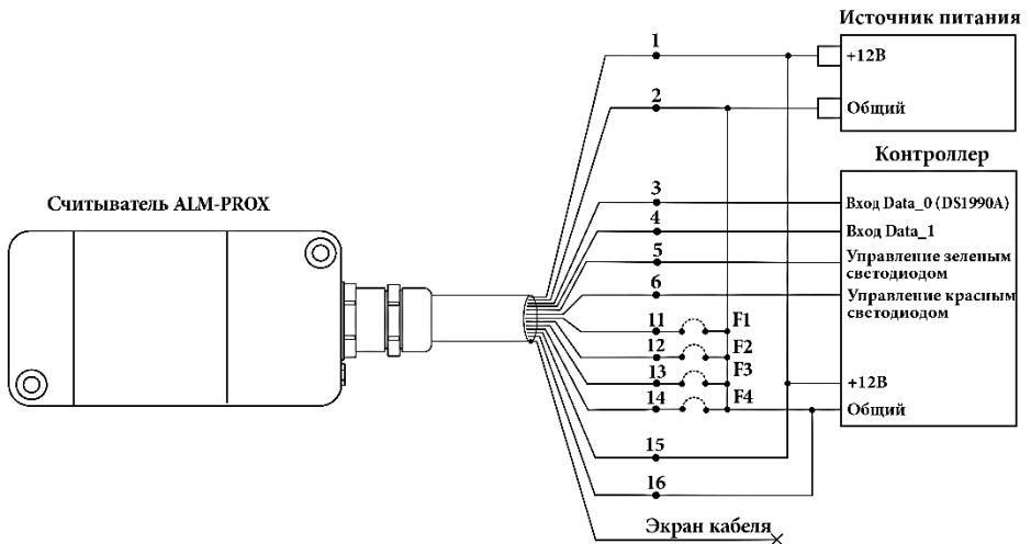
Рисунок 6 - Схема подключения счетчика ALM-PROX к контроллеру СКУД с питанием счетчика от одного источника питания.
