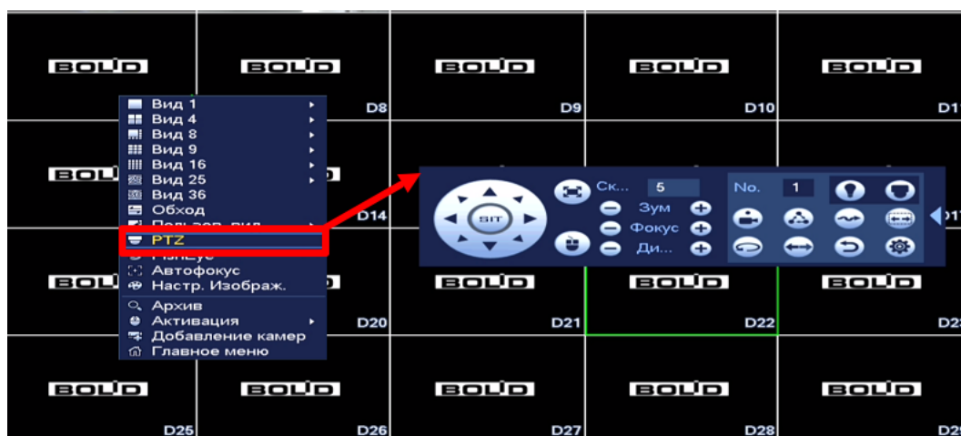
Рисунок 7.2 – Переход в меню PTZ-управления через контекстное меню
