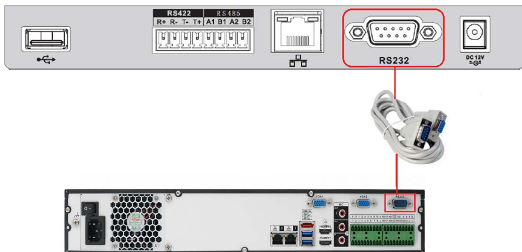
Рисунок 12.5 – Схема RS-232
