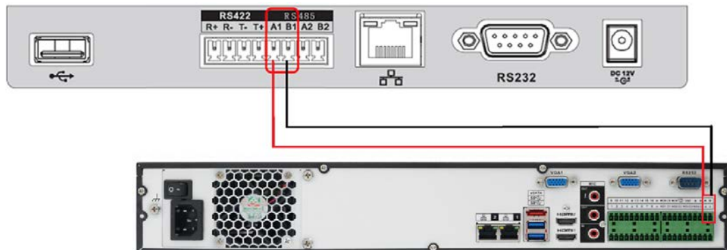
Рисунок 12.4 – Схема RS-485
