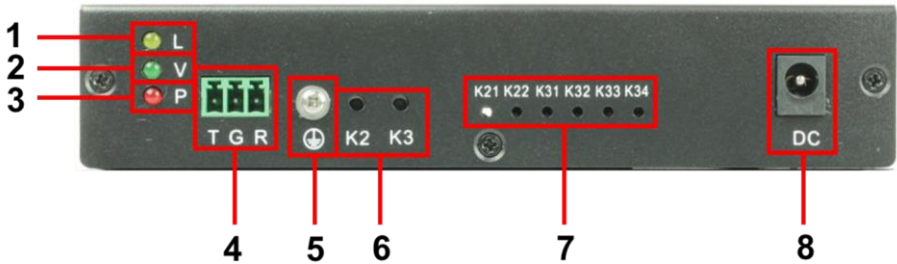
Рис.2 Передатчик TLN-NiKM2, разъемы и индикаторы на передней панели
