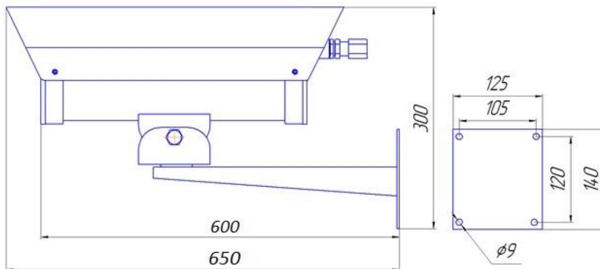
Рисунок 4.1 – Габаритные размеры термокожуха
