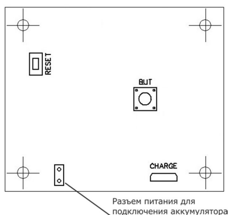
Рисунок 2. Плата радиокнопки вызова MP-413W13
