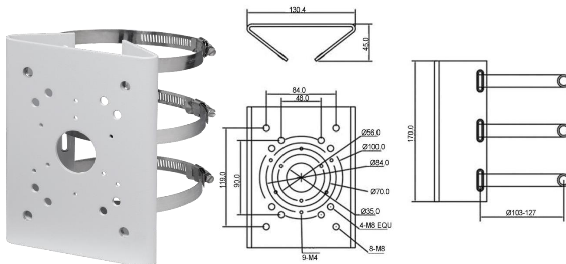
Рисунок 5.14 – Столбовой кронштейн BR-103
