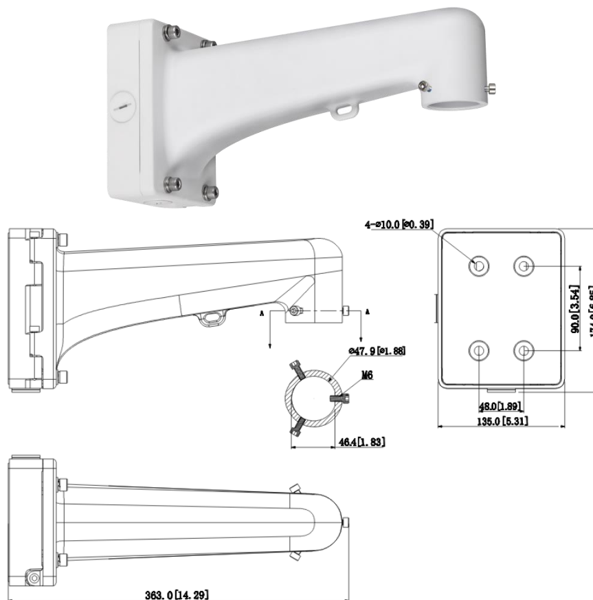
Рисунок 5.7 – Настенный кронштейн BR-110
