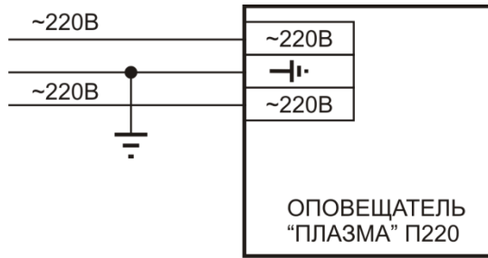
Рис.1 - Подключение оповещателя «Плазма»П220-ГОСТ к источнику питания 220В/50Гц.
